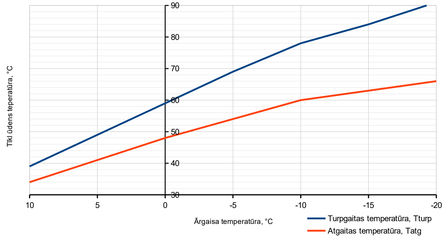
Siltumtīklu ūdens temperatūras grafiks, Bērzes ielas KM
